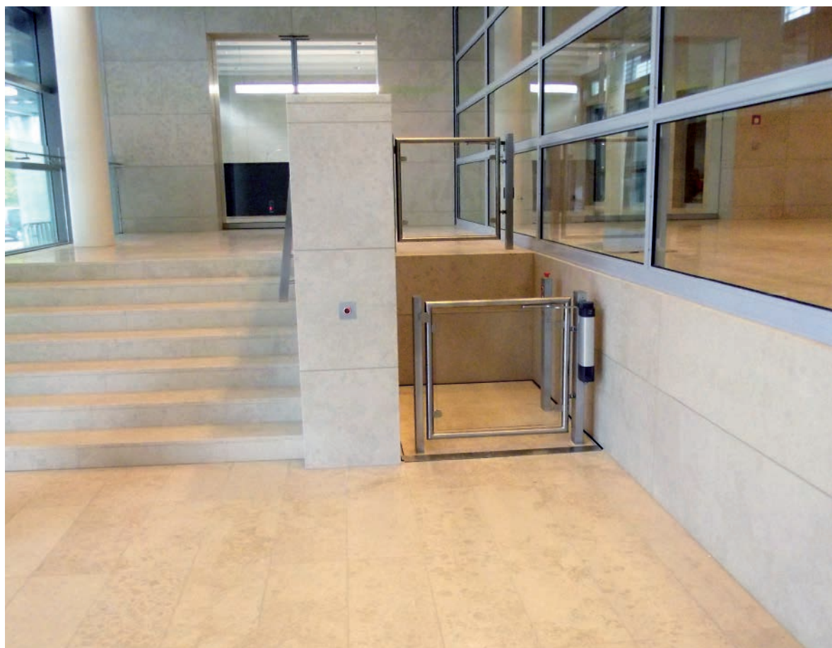
SL250 Entraînement hydraulique par système à ciseau
