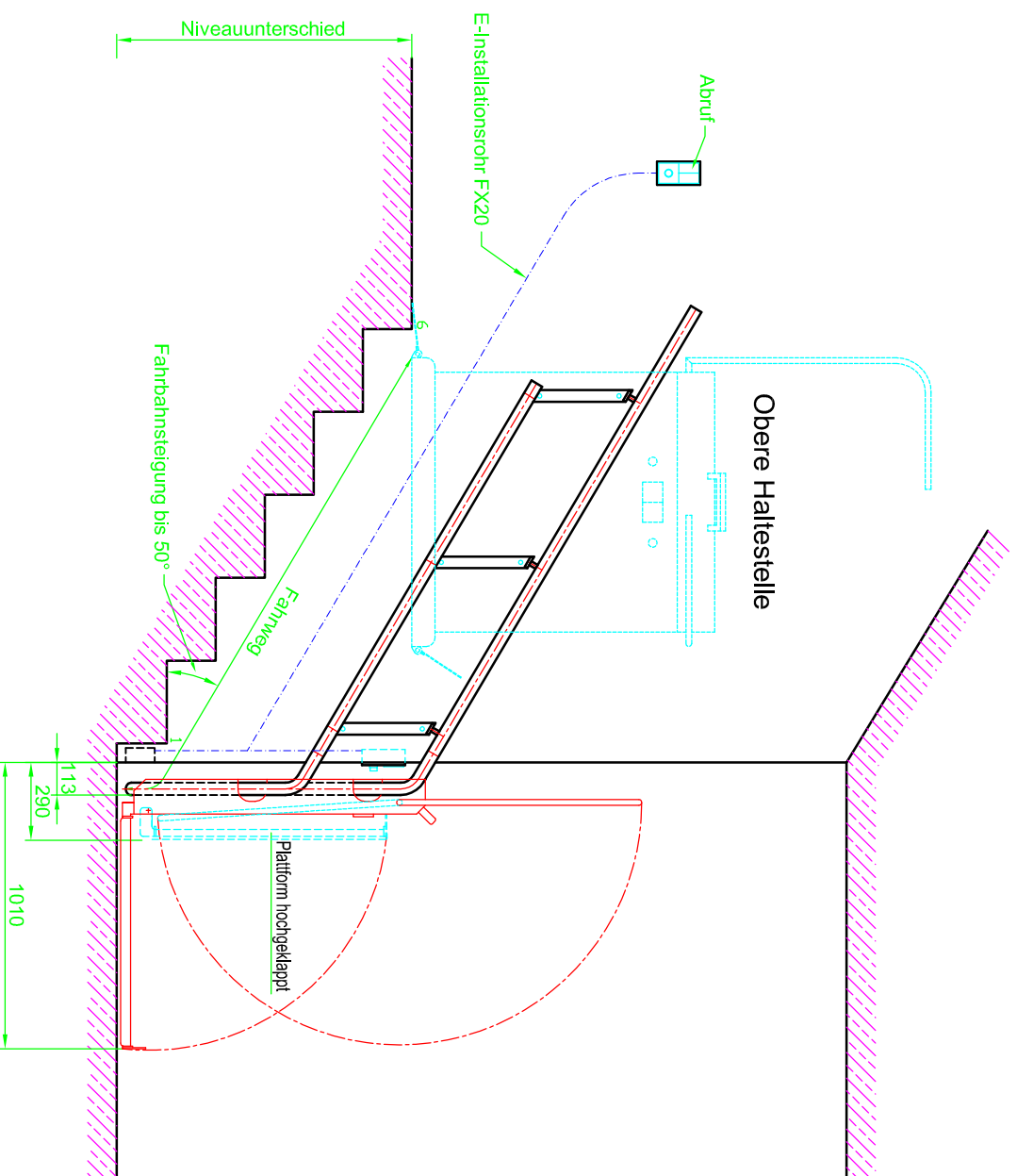
Schnitt A-B:
