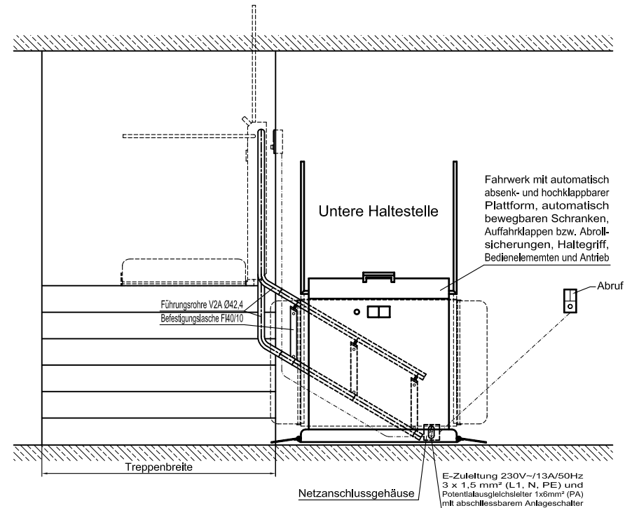
Schnitt C-D:
