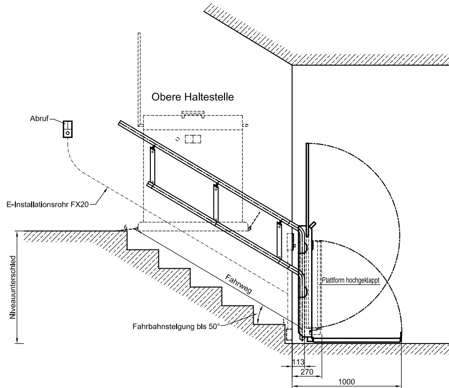
Schnitt A-B:
